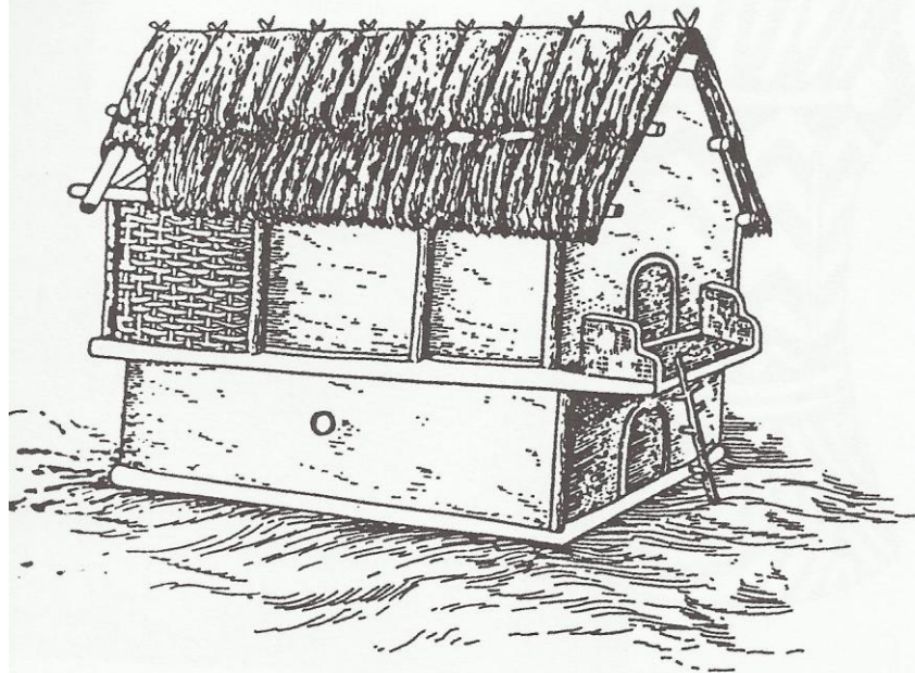
Figura 3-67 Ricostruzione ipotetica di un edificio a due piani. Insediamento di Rakovets, Ucraina occidentale. Inizio del Quarto millennio a.C.
